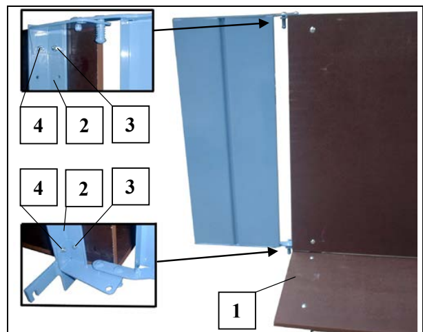
Fig. 40 Universalpritsche zusammenbauen
