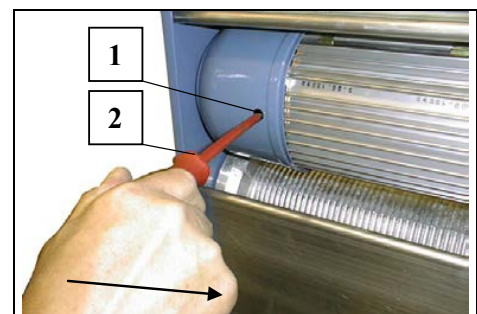
Fig. 73 Bremse lüften
