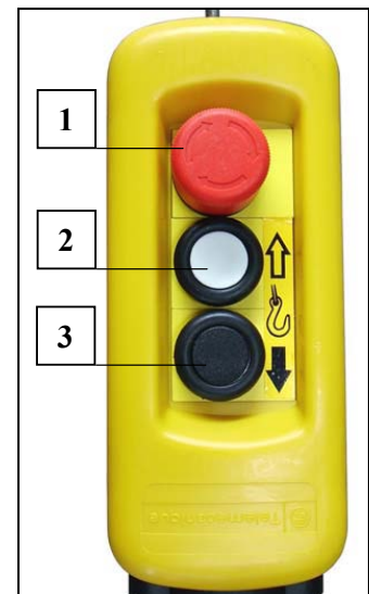
Fig. 71 Handsteuerung einstufig
