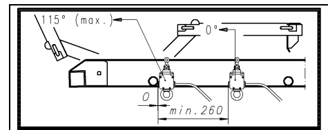
Fig. 66 PVC- Schild Endschalter
