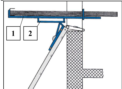
Fig. 68 Plattenpritsche mit Kippschlitten
