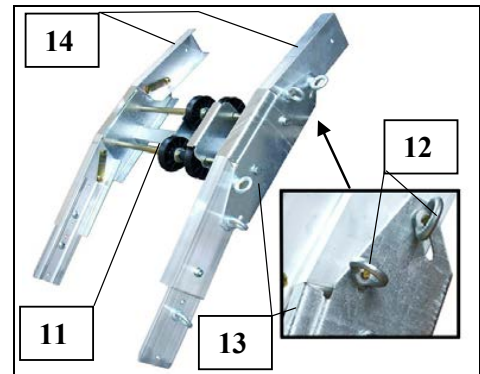
Fig. 23 Standardknickstück
