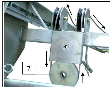
Fig. 61 Seilmontage bei Kippvorrichtung
