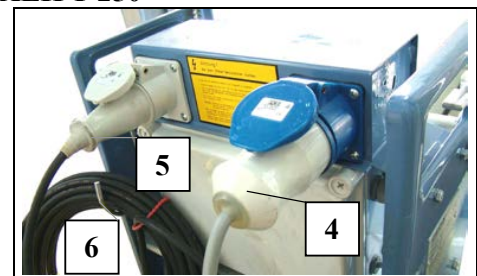
Fig. 32 Steckerleiste der Winde
