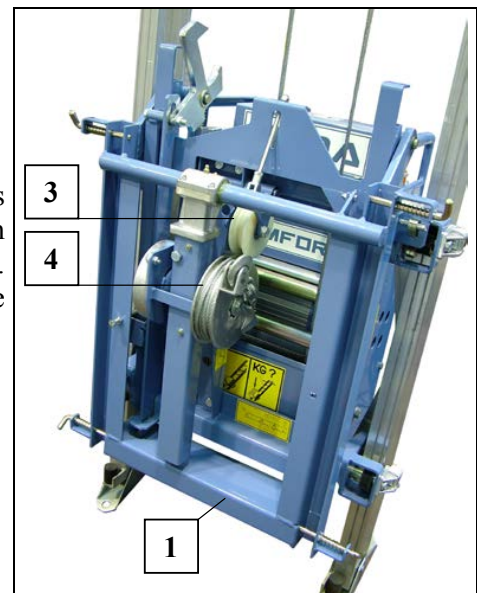
Fig. 63 Kippschlitten
