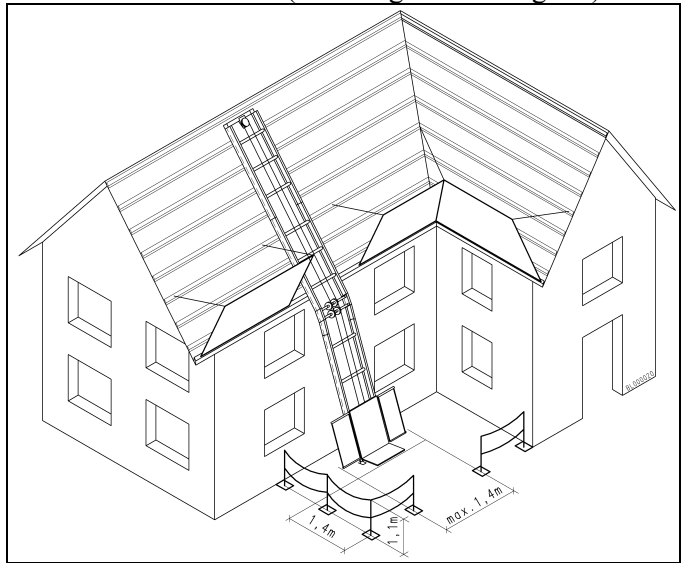
Fig. 3 Absperrung des Gefahrenbereiches
