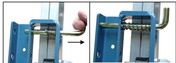
Fig. 39 Federriegel am Schlitten
