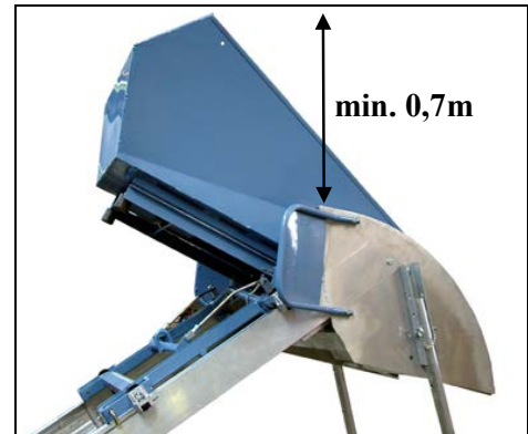
Fig. 58 Kippmulde mit Kippvorrichtung
