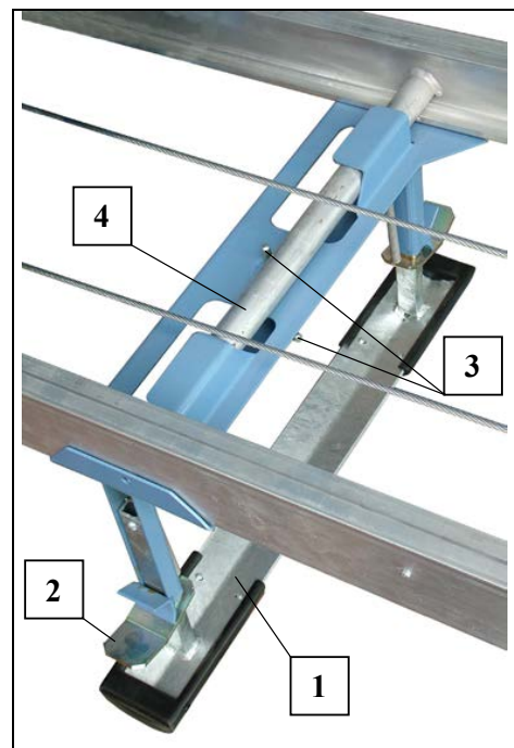
Fig. 15 Dachauflagebock
