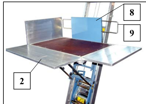
Fig. 53 Bordwände verstellen
