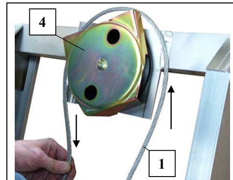
Fig. 35 Seil übers Kopfteil führen
