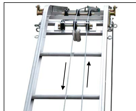
Fig. 37 Seilführung am Knickstück
