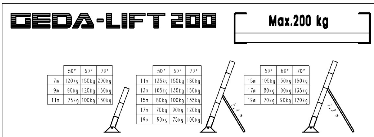
Fig. 24 Belastungstabelle für Leiterteile 150/200 kg
