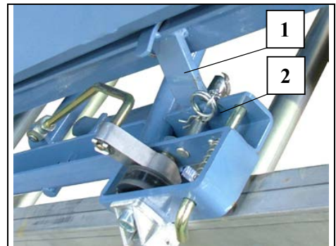
Fig. 59 Kippmulde montieren
