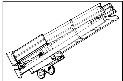
Fig. 12 Fahrgestell
