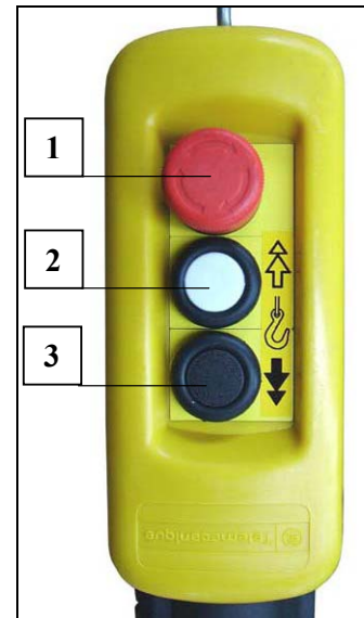
Fig. 72 Handsteuerungen zweistufig
