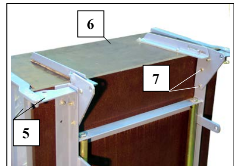
Fig. 45 Bordwand Variobühne montieren
