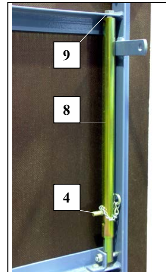
Fig. 46 Teleskopstütze Vario-Bühne
