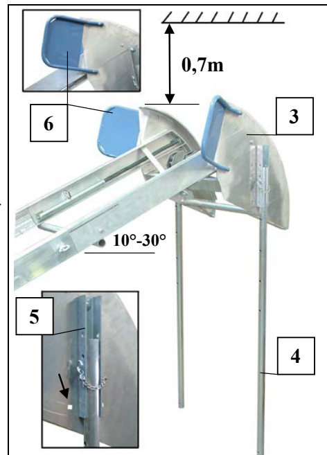
Fig. 60 Kippvorrichtung
