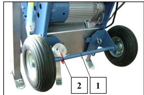
Fig. 13 Fahrgestell montieren
