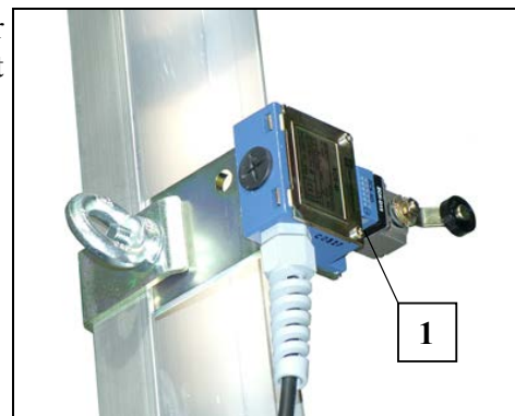
Fig. 10 Endschalter oben
