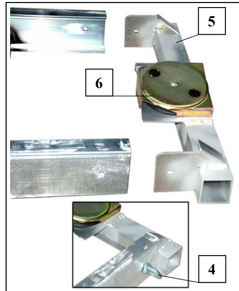
Fig. 20 Kopfstück montieren
