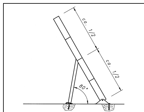
Fig. 30 Einstellwinkel der Leiterstützen
