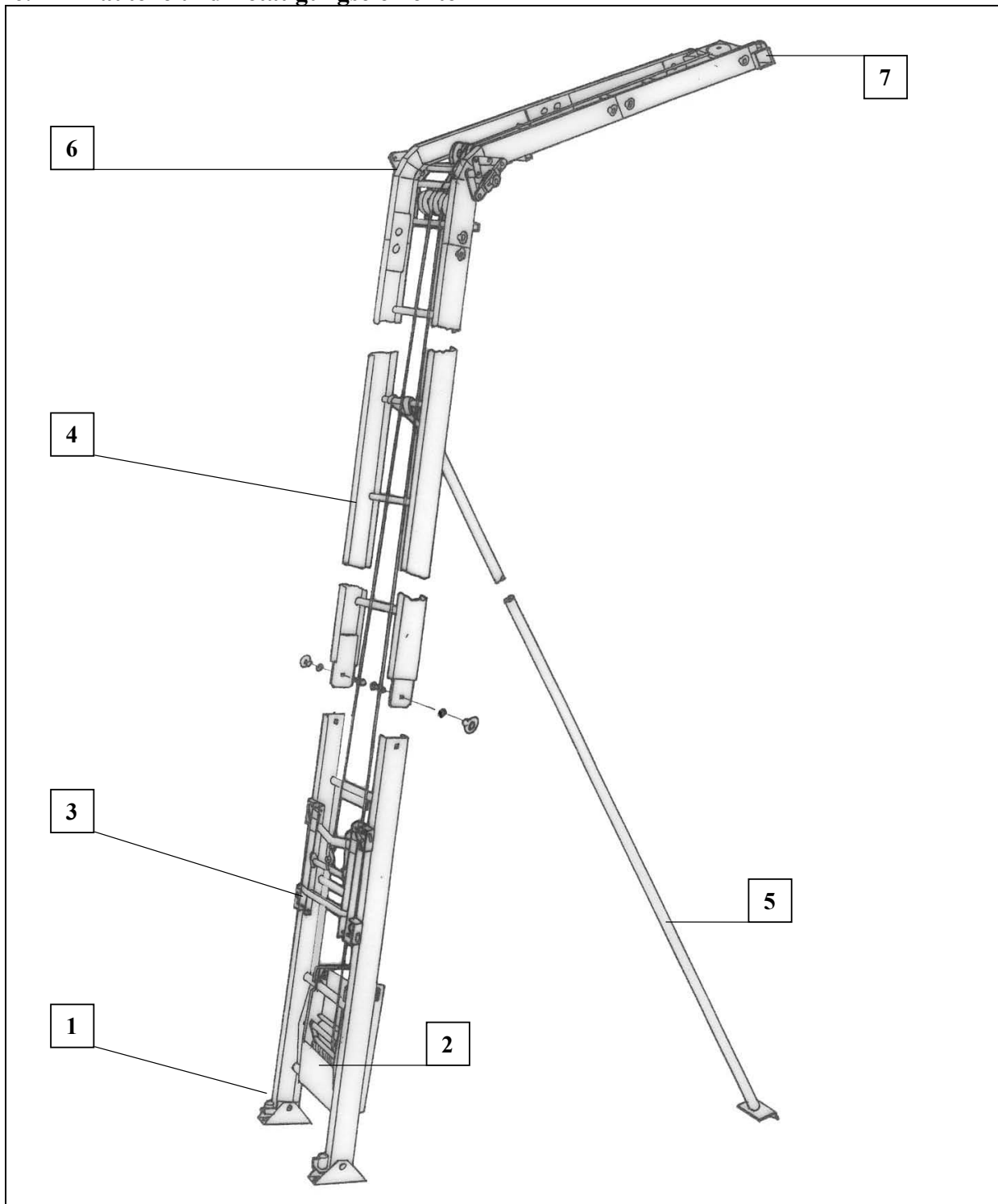
Fig. 4 GEDA-LIFT
