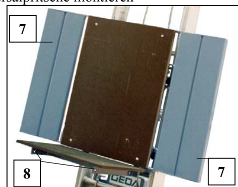
Fig. 43 Universalpritsche
