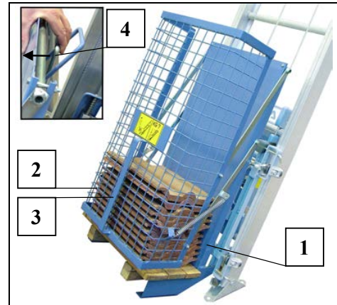
Fig. 56 Ziegelpritsche
