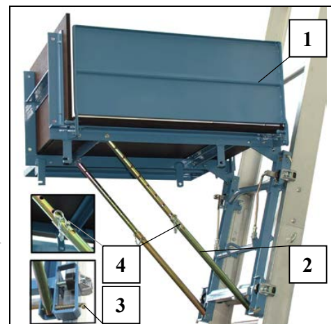
Fig. 47 Vario- Bühne
