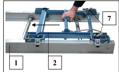
Fig. 18 Schlitten ins Fußteil einführen
