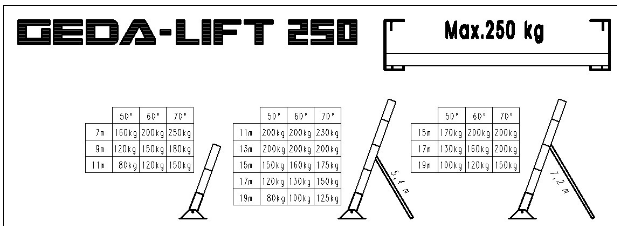
Fig. 25 Belastungstabelle für Leiterteile 200/250 kg
