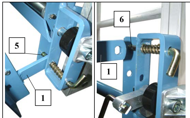
Fig. 42 Universalpritsche montieren
