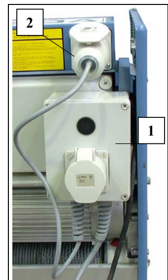
Fig. 69 Übergabesteuerung
