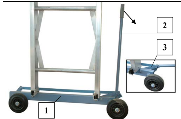
Fig. 14 Fahrwerk
