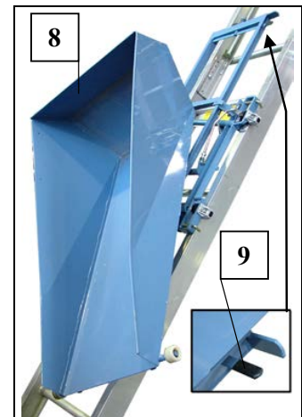
Fig. 62 Kippmulde entleeren
