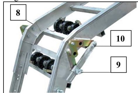
Fig. 22 Knickstück einstellen
