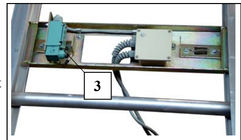
Fig. 70 Übergabeschalter
