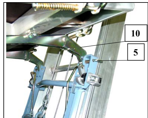
Fig. 50 Große Transportbühne montieren
