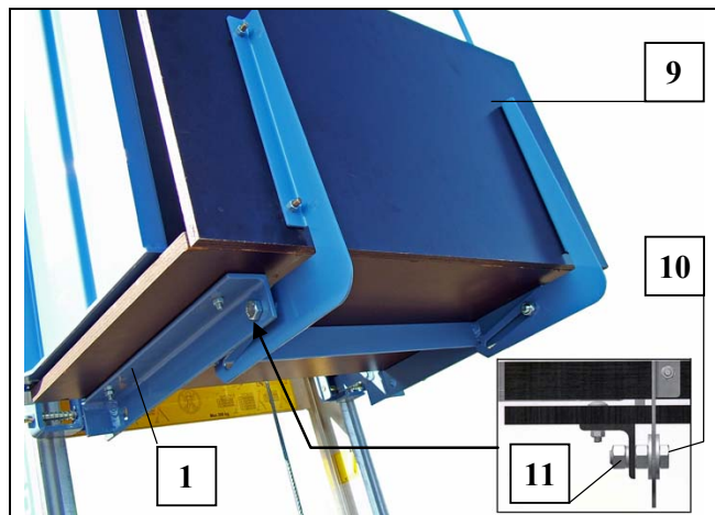
Fig. 41 Frontschutz für Universalpritsche
