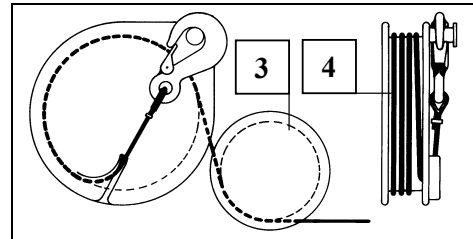
Fig. 65 PVC- Schild Seilmontage
