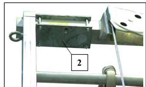
Fig. 64 Anfahrplatte am Kopfteil
