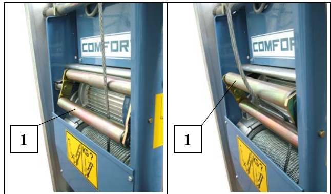
Fig. 11 Endschalter unten
