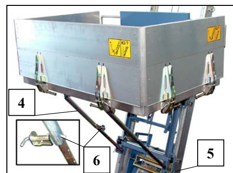
Fig. 51 Transportbühne
