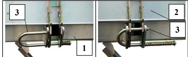
Fig. 49 Bordwände der Transportbühne montieren
