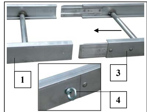
Fig. 19 Leiterteile zusammenbauen
