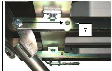
Fig. 52 Teleskopstützen abstecken
