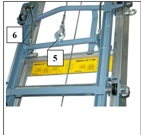
Fig. 38 Seil am Schlitten einhängen
