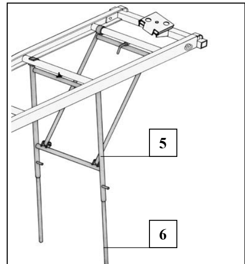
Fig. 55 Abstützung für Leiterbahn
