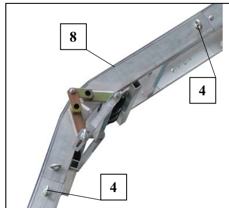
Fig. 21 Knickstück montieren
