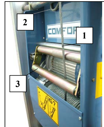
Fig. 34 Seil abspulen
