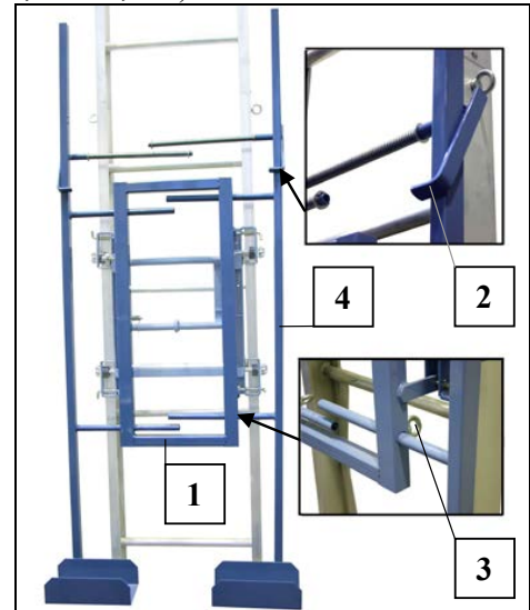
Fig. 54 Plattenpritsche
