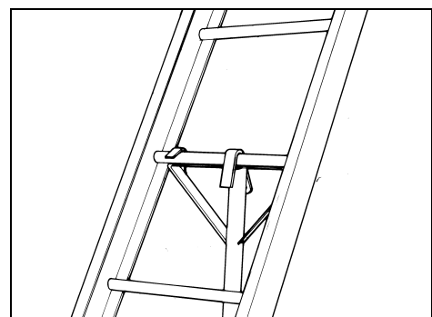
Fig. 28 Alu-Leiterstütze einhängen
