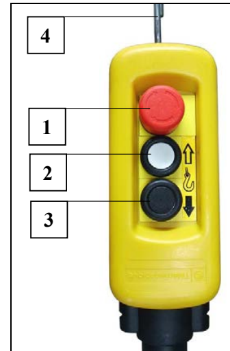
Fig. 8 Handsteuerung (1-stufig)
