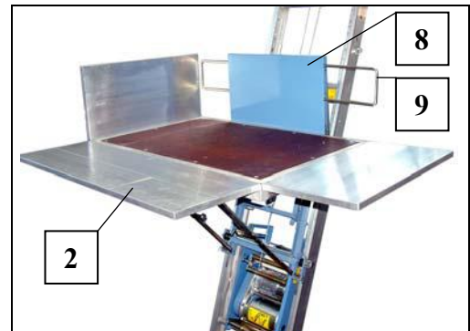
Fig. 53 Bordwände verstellen
