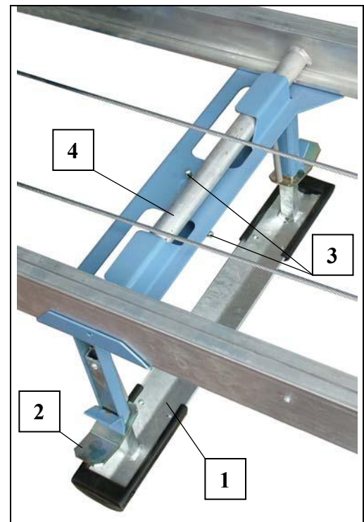
Fig. 15 Dachauflagebock
