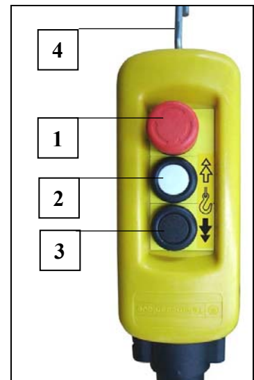
Fig. 9 Handsteuerung (2-stufig)
