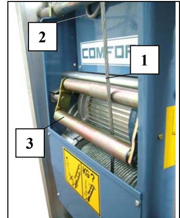
Fig. 34 Seil abspulen
