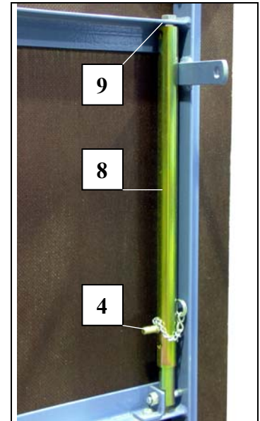
Fig. 46 Teleskopstütze Vario-Bühne
