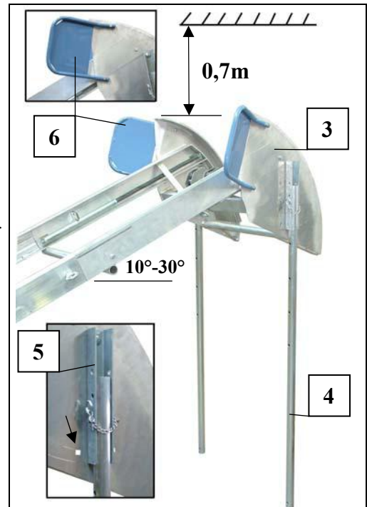
Fig. 60 Kippvorrichtung
