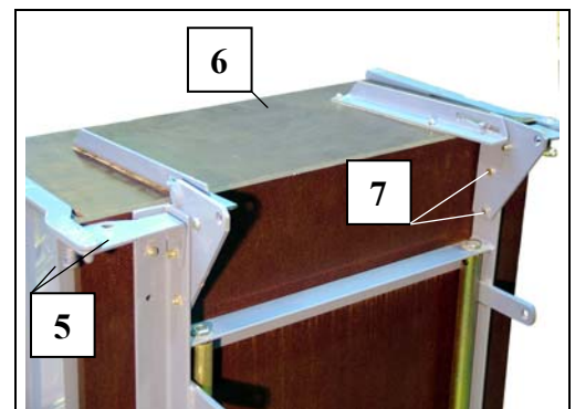
Fig. 45 Bordwand Variobühne montieren
