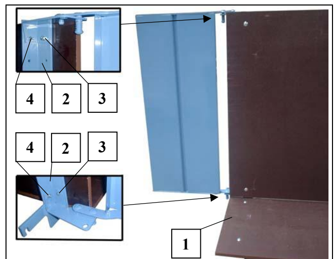
Fig. 40 Universalpritsche zusammenbauen
