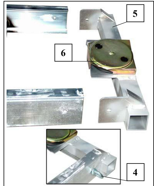
Fig. 20 Kopfstück montieren
