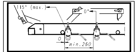
Fig. 66 PVC- Schild Endschalter
