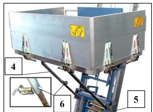
Fig. 51 Transportbühne
