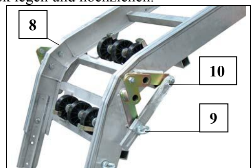
Fig. 22 Knickstück einstellen
