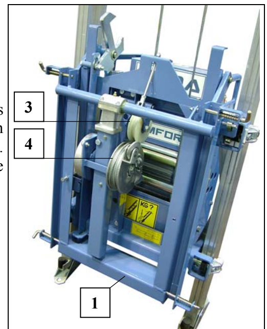
Fig. 63 Kippschlitten
