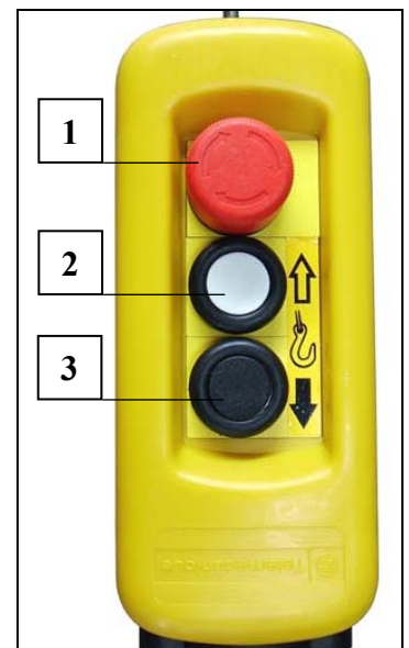
Fig. 71 Handsteuerung einstufig
