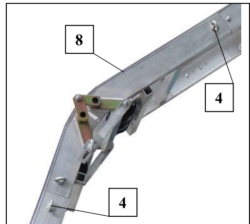
Fig. 21 Knickstück montieren
