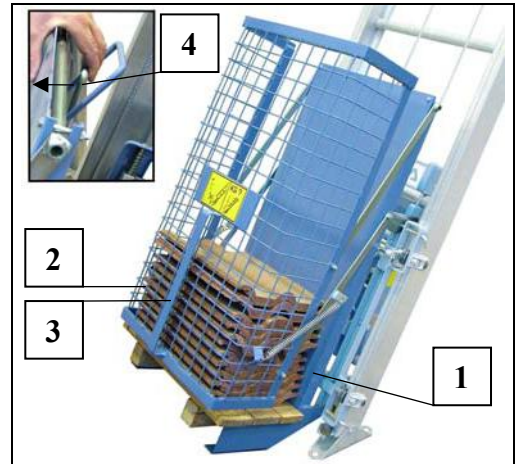
Fig. 56 Ziegelpritsche
