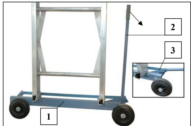
Fig. 14 Fahrwerk
