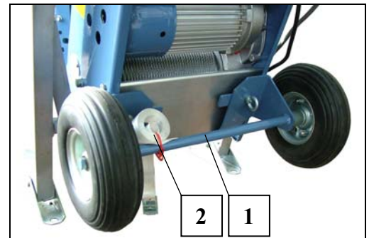
Fig. 13 Fahrgestell montieren
