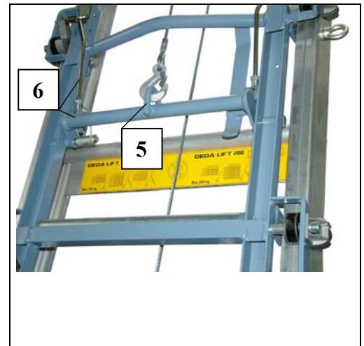
Fig. 38 Seil am Schlitten einhängen
