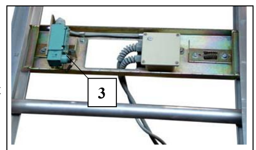
Fig. 70 Übergabeschalter
