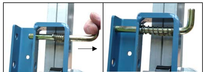
Fig. 39 Federriegel am Schlitten
