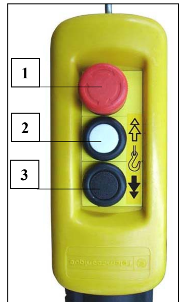
Fig. 72 Handsteuerungen zweistufig
