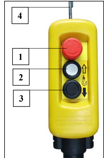
Fig. 8 Handsteuerung (1-stufig)
