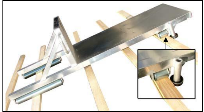
Fig. 16 Dachziegelverteiler
