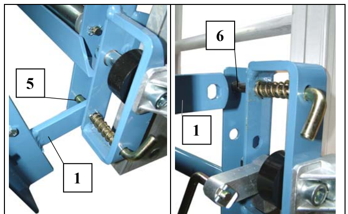
Fig. 42 Universalpritsche montieren
