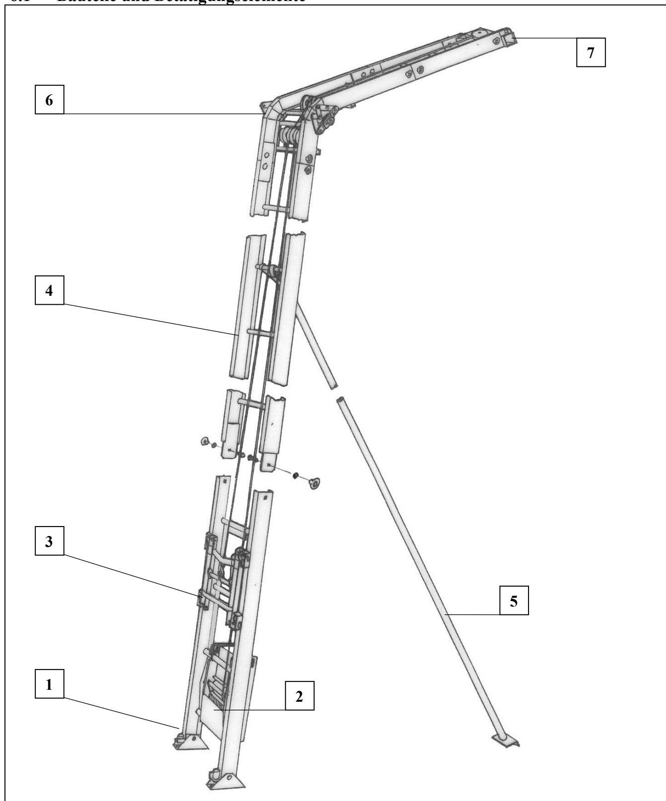
Fig. 4 GEDA-LIFT
