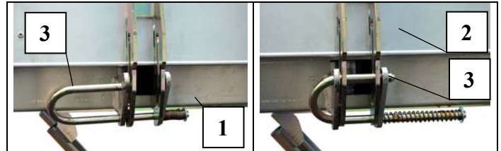
Fig. 49 Bordwände der Transportbühne montieren
