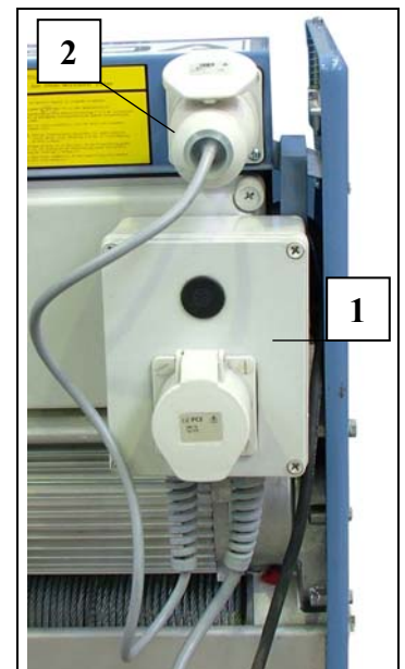
Fig. 69 Übergabesteuerung
