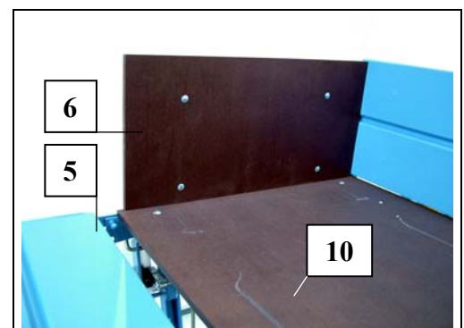
Fig. 48 Bordwand und Seitenschutz abklappen
