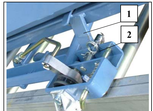
Fig. 59 Kippmulde montieren
