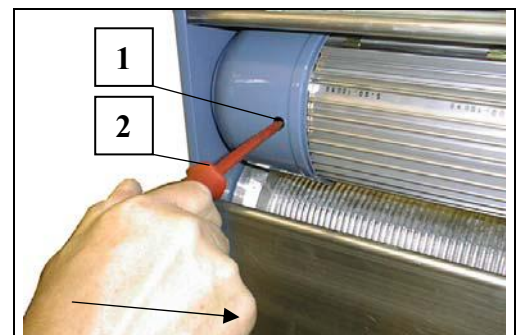
Fig. 73 Bremse lüften
