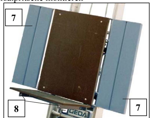
Fig. 43 Universalpritsche
