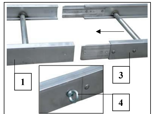
Fig. 19 Leiterteile zusammenbauen
