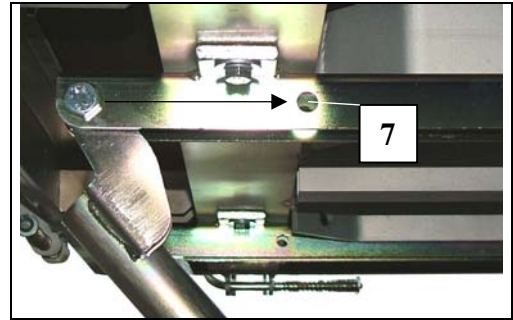
Fig. 52 Teleskopstützen abstecken
