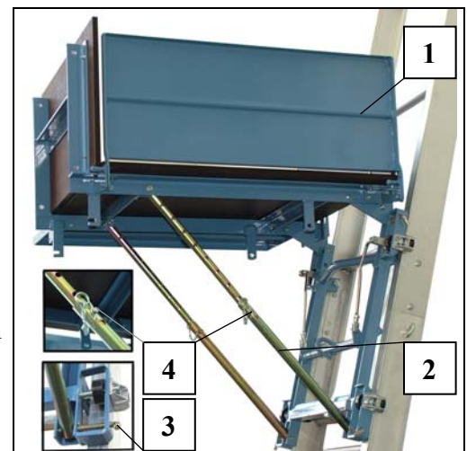
Fig. 47 Vario- Bühne
