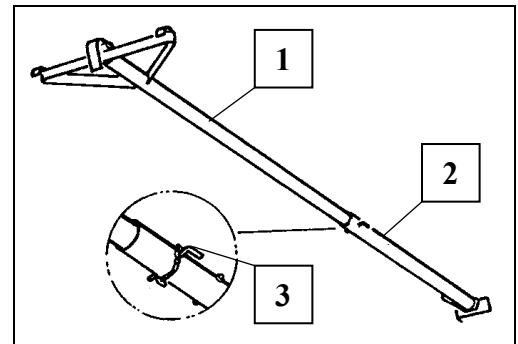
Fig. 27 Alu-Leiterstütze
