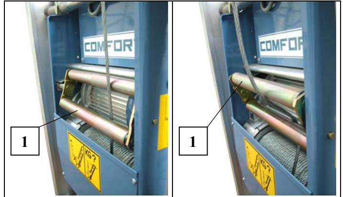
Fig. 11 Endschalter unten
