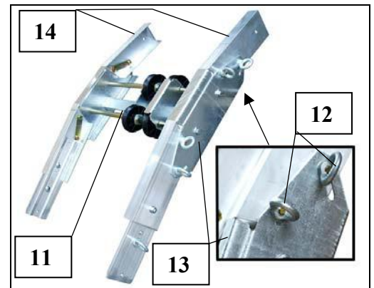
Fig. 23 Standardknickstück
